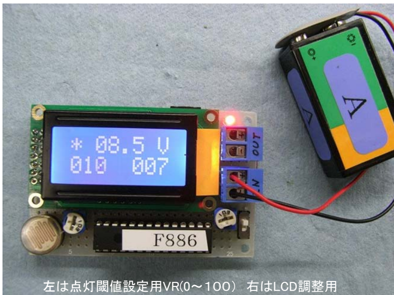
LCD 2行目左の現在の暗さ(0~100)数値が、右の設定値(0~100)を上回ると点灯する
